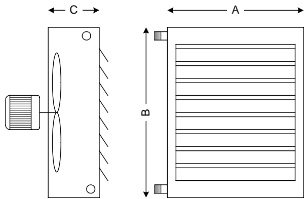
Modèle 1 rangée / Diffuseur de type volets
