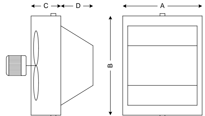
Modèle 2 rangées / Diffuseur de type convergent
